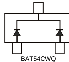
BAT54CWQ
